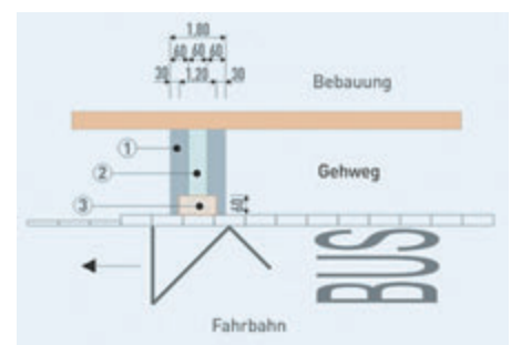
Bild 7: Verlegung von Bodenindikatoren an einer Bushaltestelle
