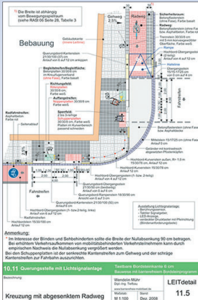
Bild 8: Detailzeichnung einer Kreuzung mit abgesenktem Radweg als „LEITdetail“ gekennzeichnet
