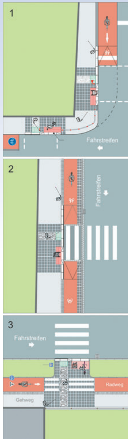
Bild 3: Querungsstellen mit Entschärfung Fußgängerübergang zum baulichen Radweg
