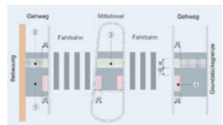
Bild 6: Verlegung von Bodenindikatoren an einer getrennten Querungsstelle
